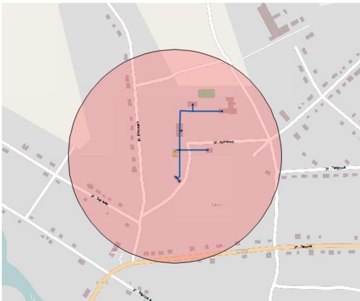
Рисунок 3. Радиус эффективного теплоснабжения от котельной МУП «Еланское ЖКХ»
