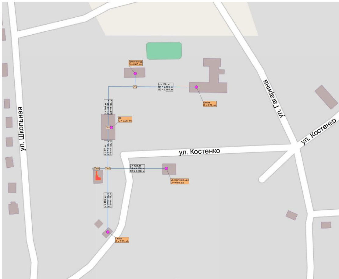
Рисунок 5. Тепловые сети от котельной МУП «Еланское ЖКХ»
