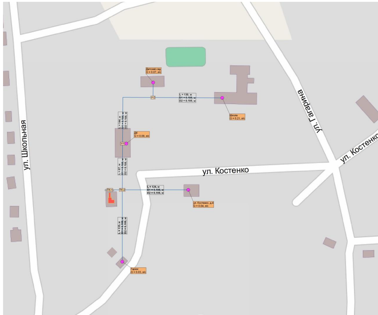
Рисунок 2. Зона действия котельной МУП «Еланское ЖКХ» (расчетная схема)
