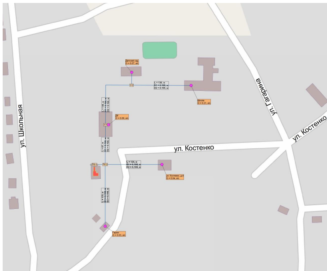
Рисунок 4. Зона действия котельной МУП «Еланское ЖКХ»
