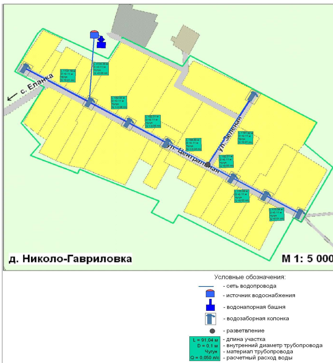
Рисунок 6 - Существующая схема водопроводной сети д. Николо-Гавриловка
