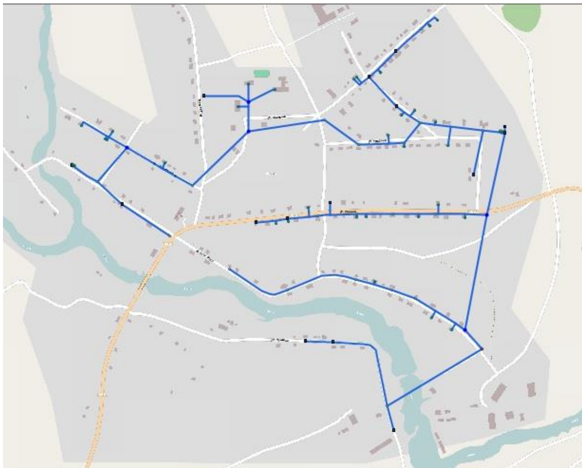
Рисунок 9 - Существующая схема водопроводной сети с. Еланка
