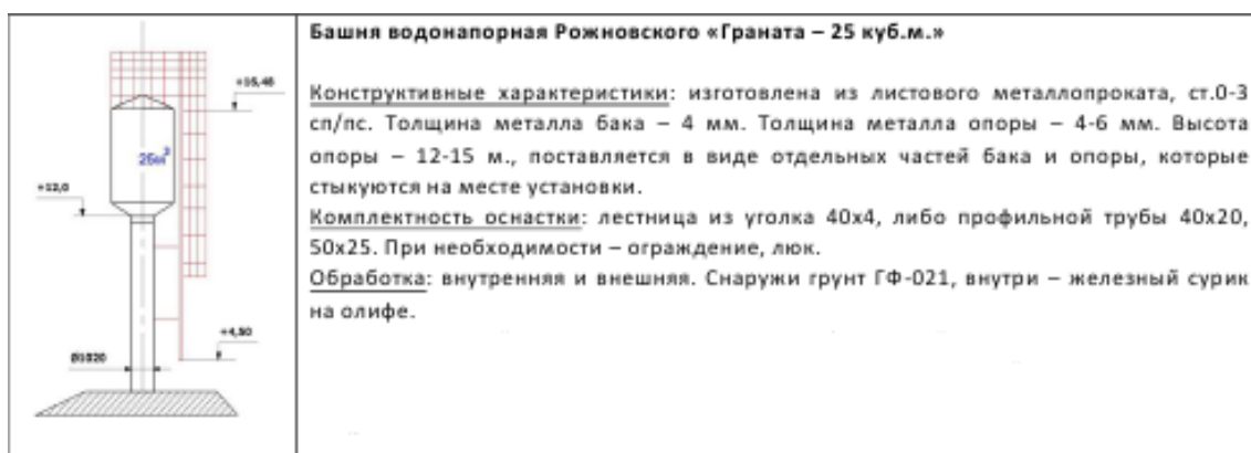
Рисунок 8 - Основные характеристики водонапорной башни
