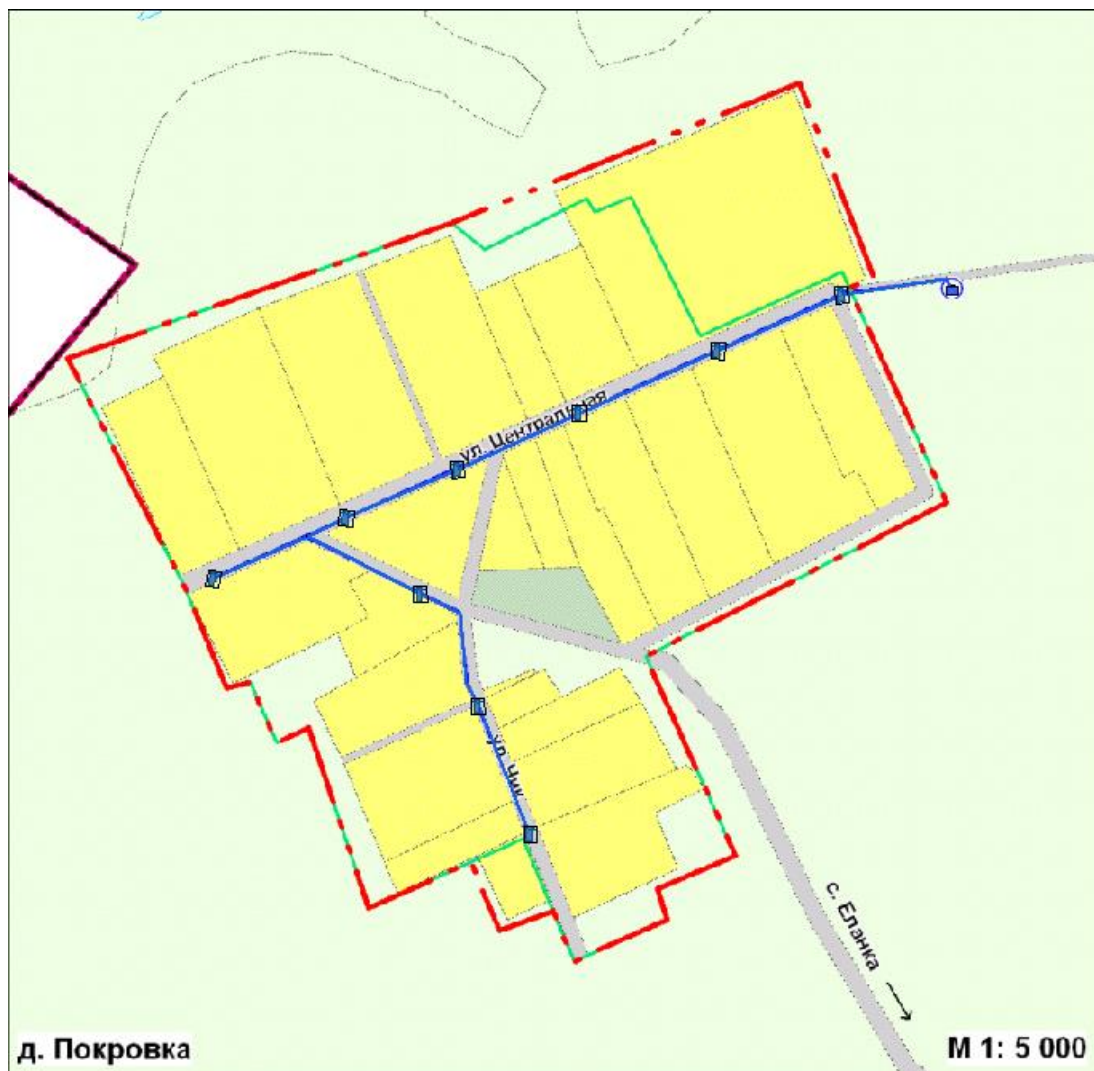
Рисунок 6 - Существующая схема водопроводной сети д. Покровка
