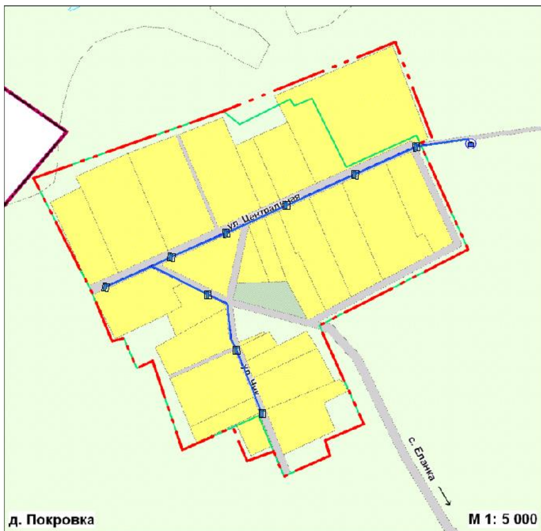
Рисунок 1 - Зона действия централизованного водоснабжения д. Покровка
